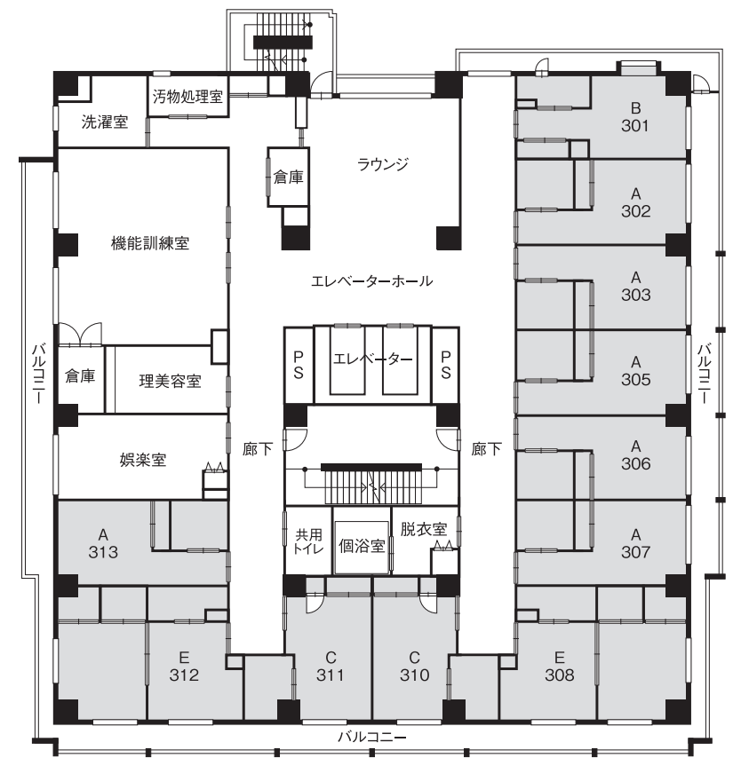
3階平面図
