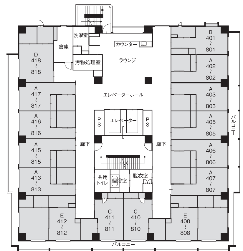
4～8階平面図
